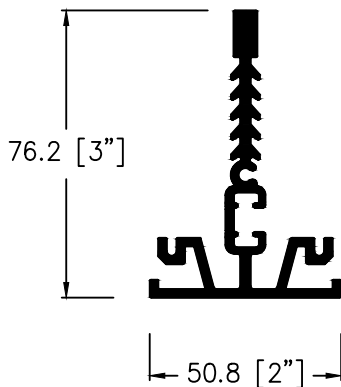
3030 3" T-BAR
