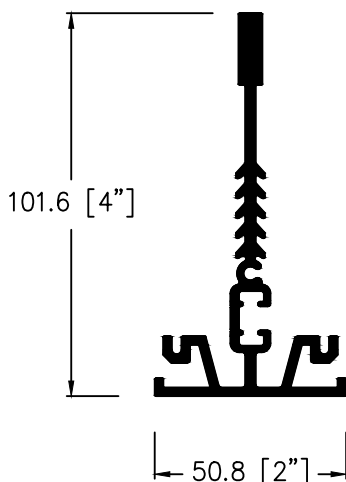
3040 4" T-BAR
