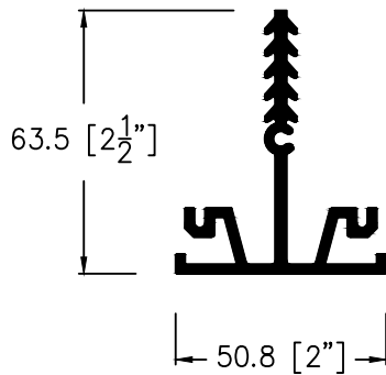
3025 2 1/2" T-BAR
