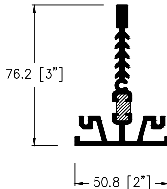
3035 3" T-BAR
