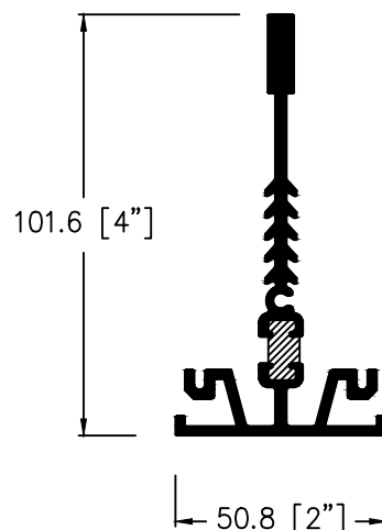
3045 4" T-BAR
